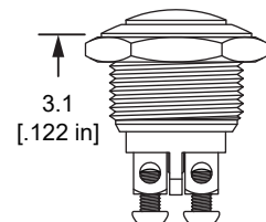
Domed Actuator
